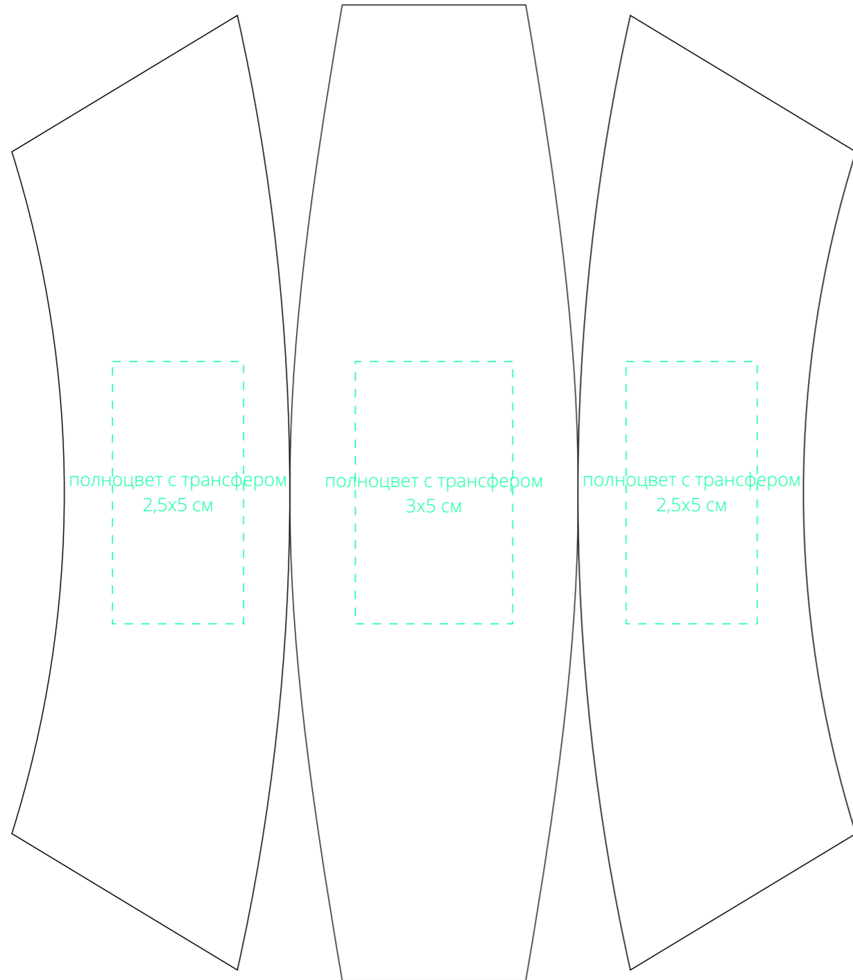
панели M1:1
