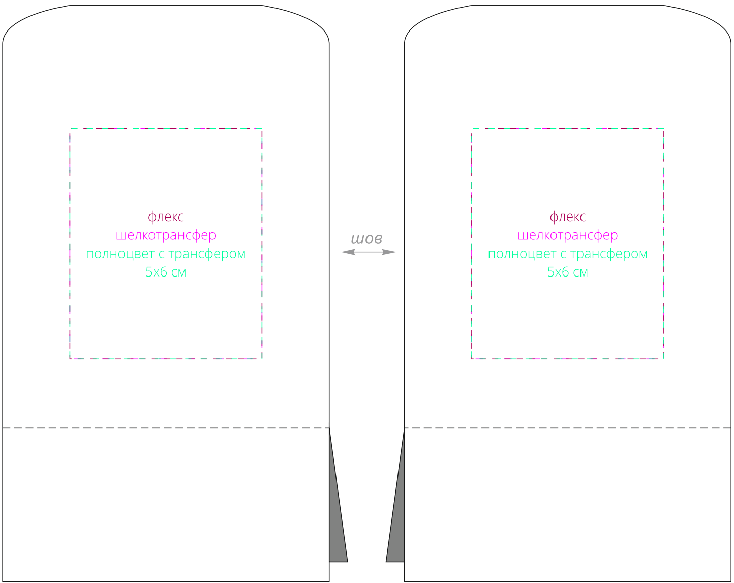
чехол M1:1
