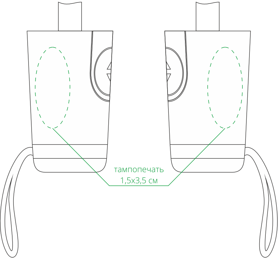
ручка M1:1
